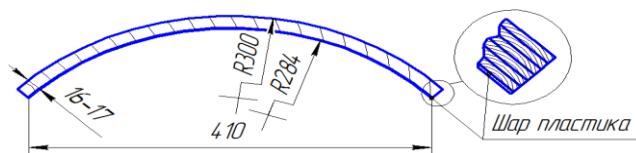
Зовнішній радіус
